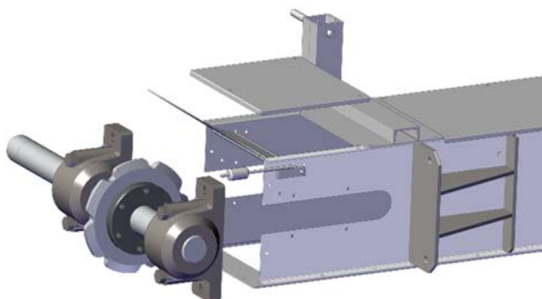
Tourteau démontable par l'arrière
