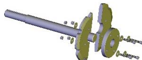
Tourteau démontable
